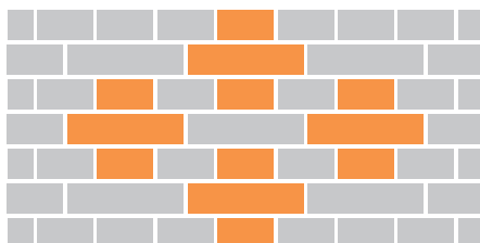
Polokřížová väzba
