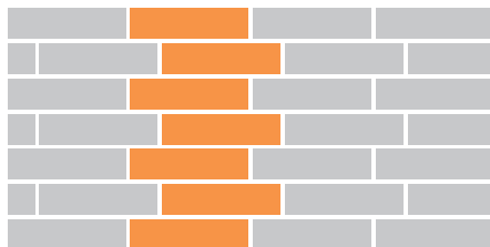
Behúňová väzba trojštvrťová zvislá
