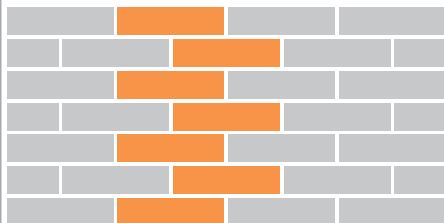
Behúňová väzba polovičná
