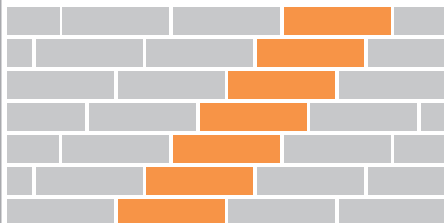
Behúňová väzba trojštvrťová šikmá
