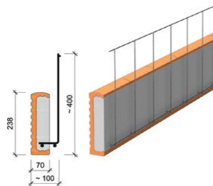
Porotherm KP Vario 200 až 350 nosný železobetónový diel
