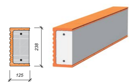
Porotherm KP Vario 100 až 175 nosný železobetónový diel
